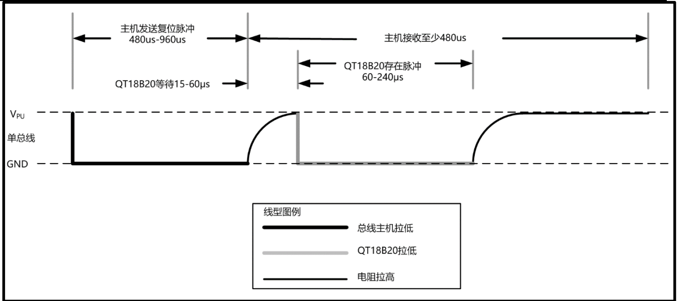
图 13 初始化时序
