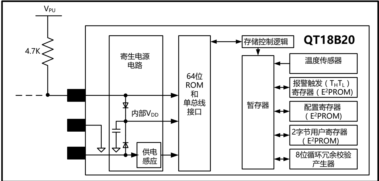
图 1 QT18B20 框图
