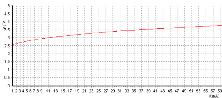
电流-电压曲线 Current-Voltage Curve
