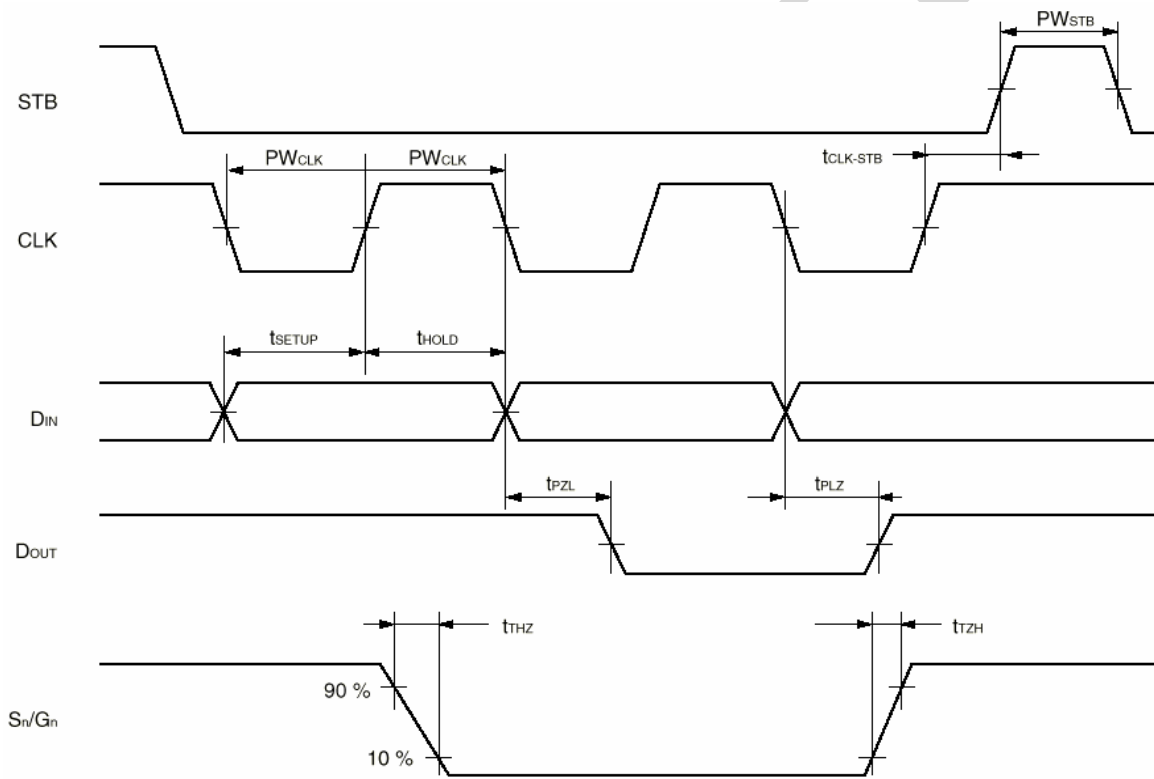
时序波形图:
