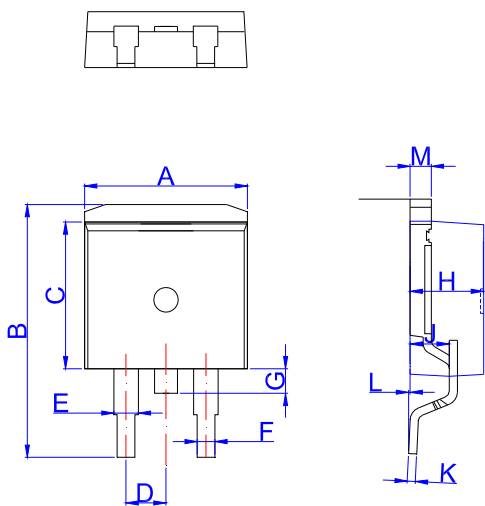
TO-263
