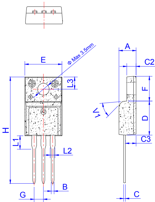
TO-220F Ins
