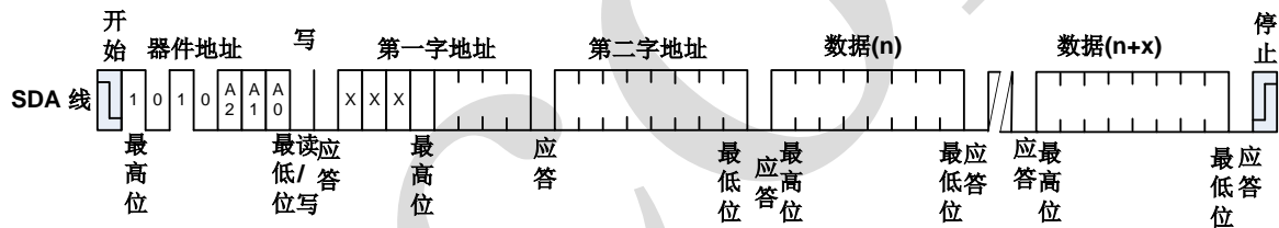
图 9、页写
