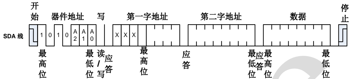
图 8、字节写
