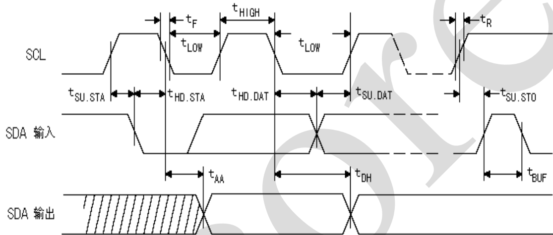
图 5、总线时序
