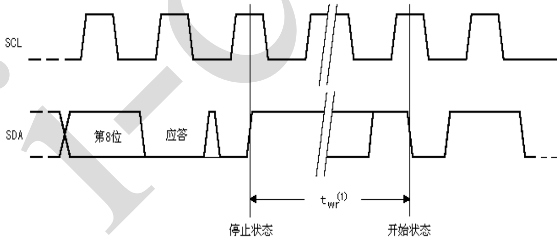
图 5、总线时序
