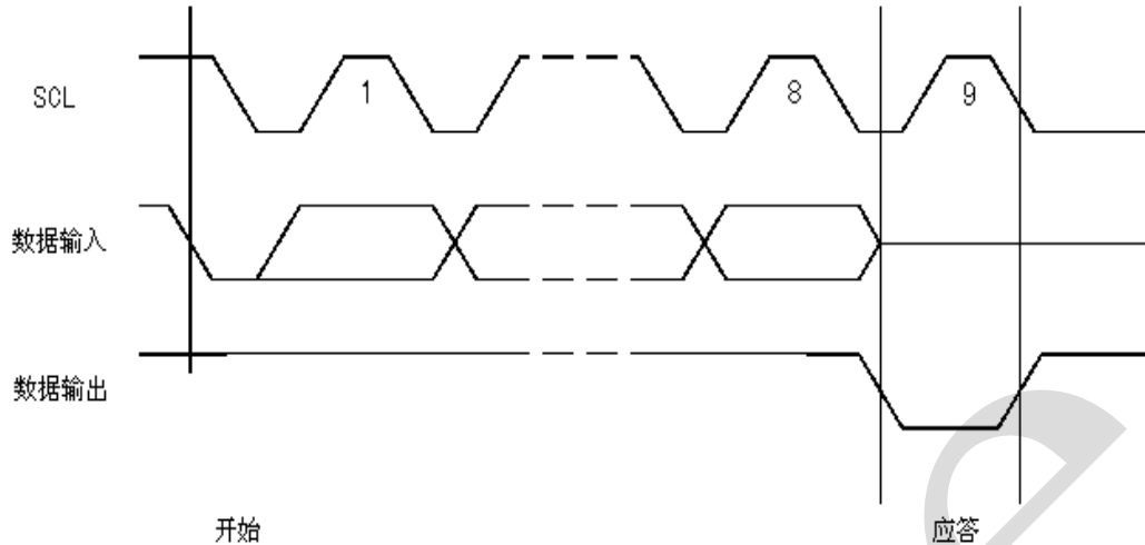
图 7、输出响应
