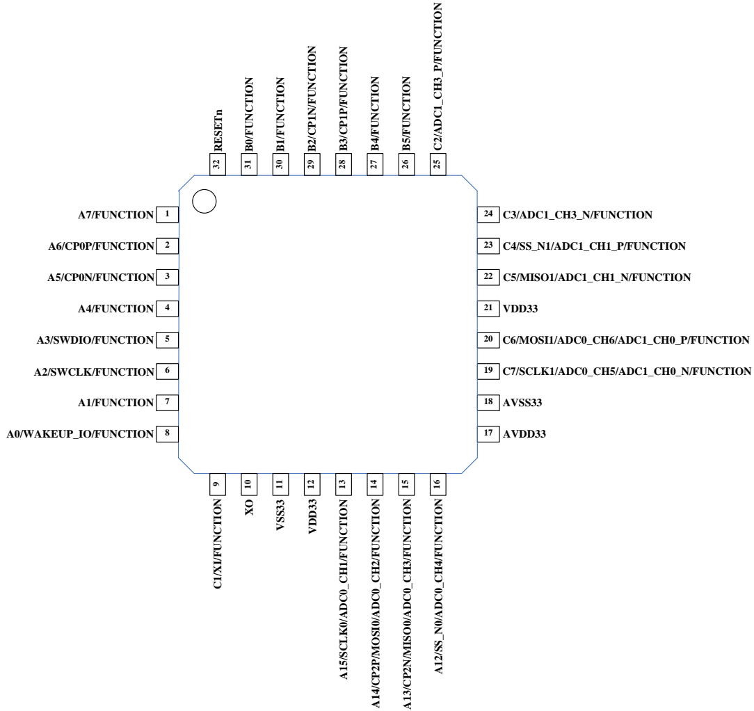
图 5-1KCT6 封装管脚配置
