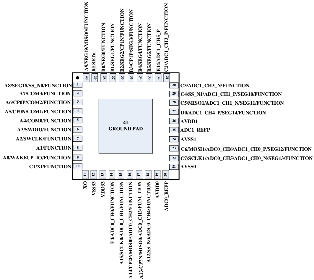
图 5-2 DBU6 封装管脚配置
