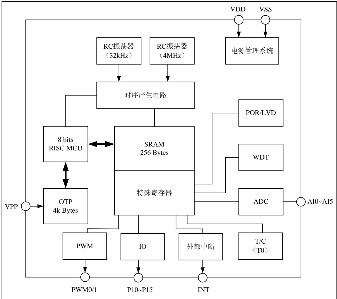
图2. 功能框图
