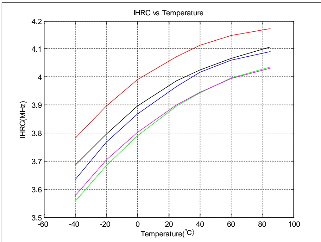
图 6. IHRC 温度特性曲线
