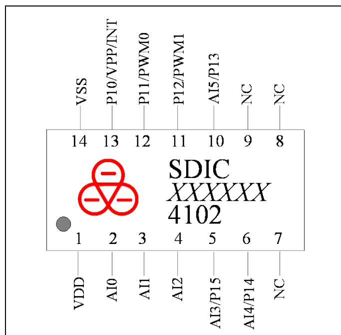
图1. 管脚图
