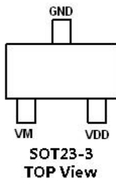
图二、引脚配置
