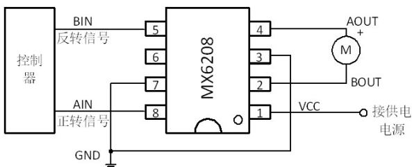
典型应用图
