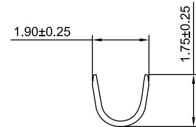
SEC:B-B
